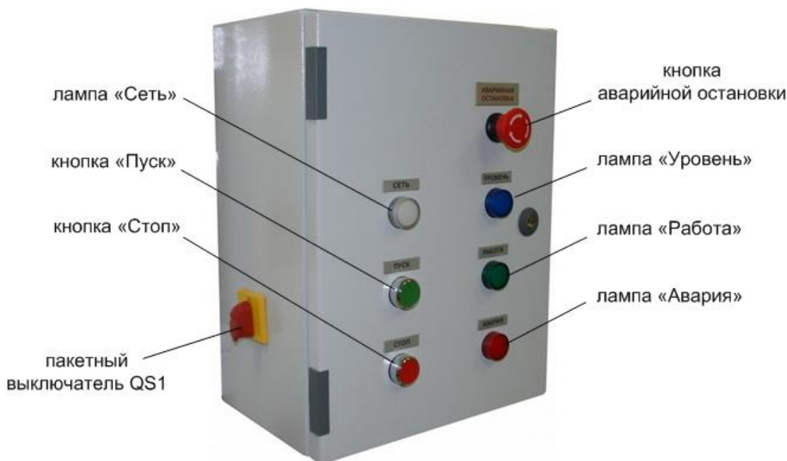
Рис.4 Блок управления.
