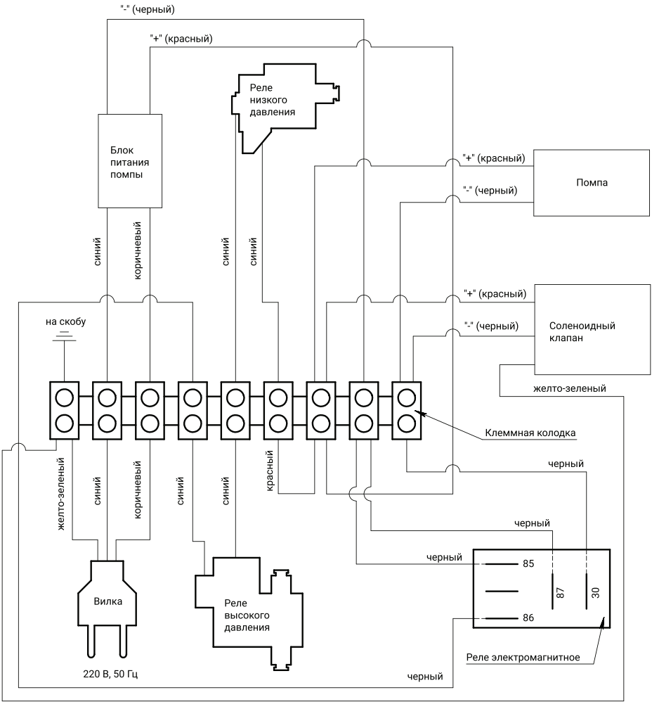
Рис. 13 Электрическая схема.
