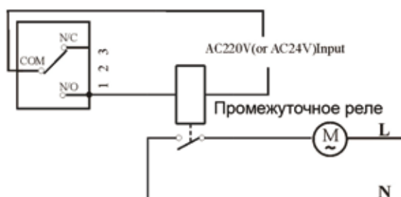
Управление повышающим насосом через промежуточное реле (ток>5А)
