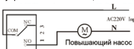
Прямое управление повышающим насосом (ток<5А)
