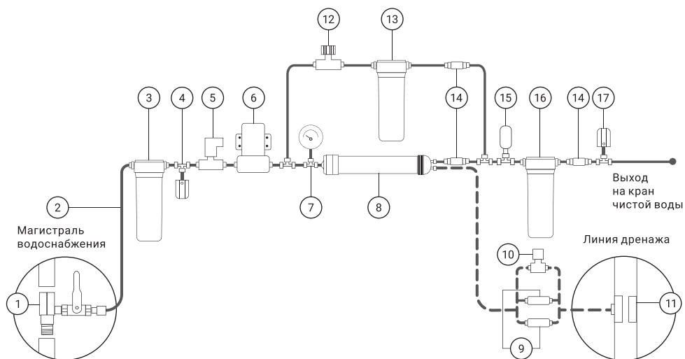
Рис. 1. Схема подключения Гейзер Presto.
