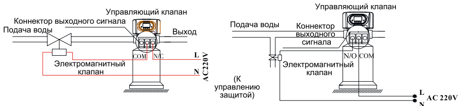
Рис. 3-2 Цепь управления электромагнитным клапаном на входе
