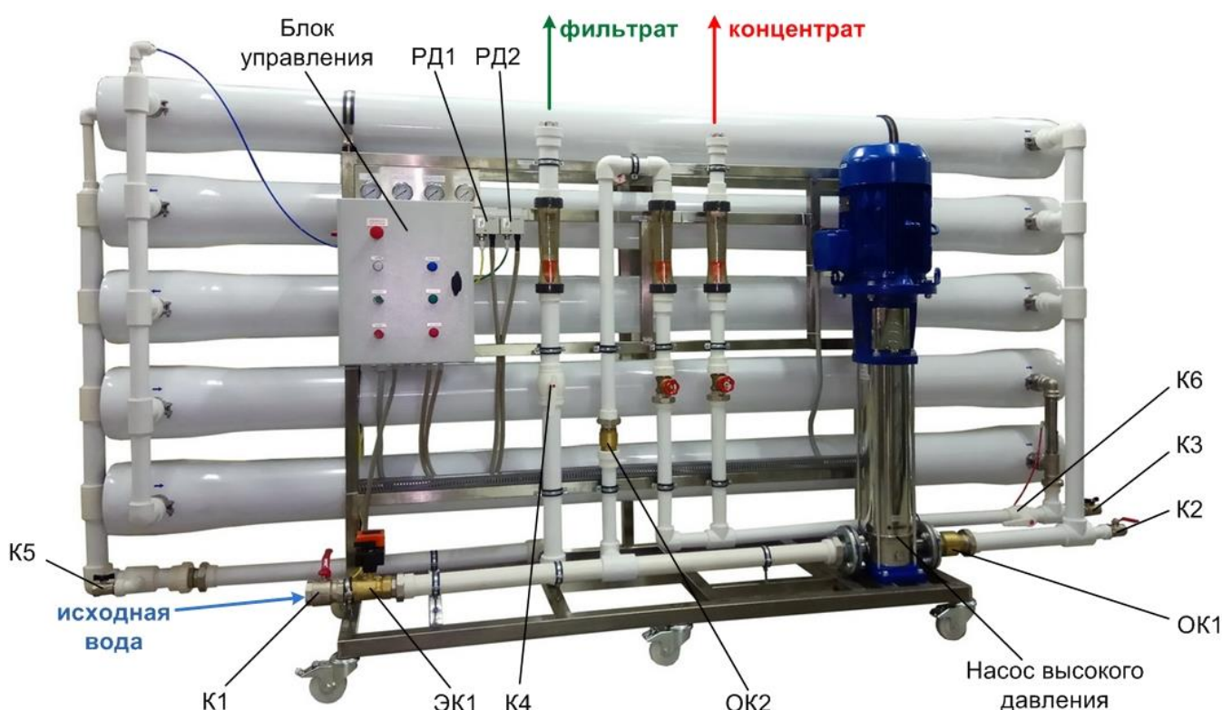
Рис.1 Общий вид установки.
