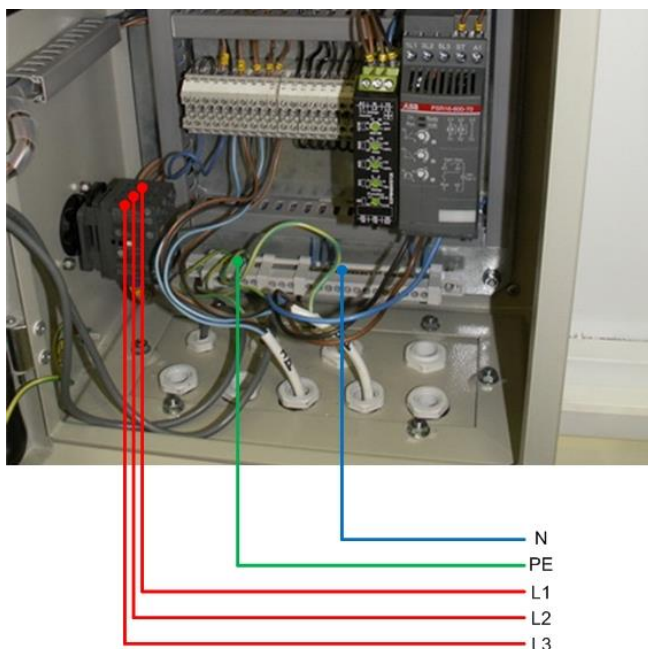
Рис.7 Подключение электропитания.
