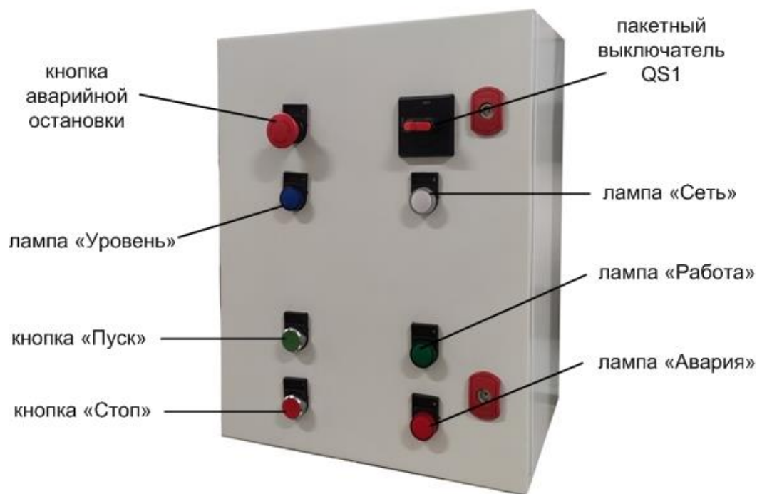
Рис.4 Блок управления.
