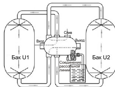
Бак U1 в рабочем режиме, бак U2 в режиме обратной промывки
