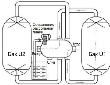
Бак U1 в рабочем режиме, бак U2 в ждушем режиме
