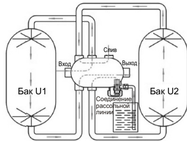
Бак U2 в рабочем режиме, бак U1 в режиме солевой и медленной промывки (регенерация нисходящим потоком)
