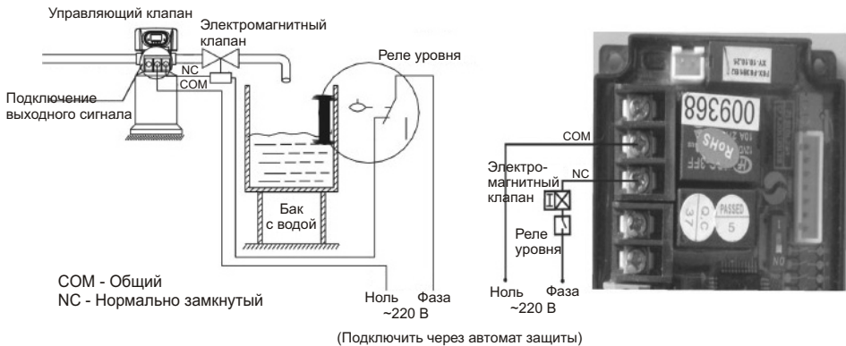
Рисунок 3-2. Подключение электромагнитного клапана на выходе
