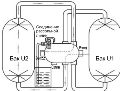
Бак U2 в рабочем режиме, бак U1 в режиме опускания смолы
