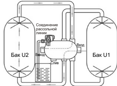
Бак U2 в рабочем режиме, бак U1 в ждушем режиме
