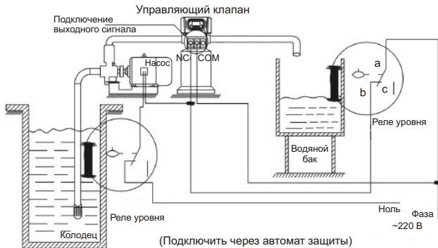
Рисунок 3-5. Подключение регулятора уровня для управления входным насосом
