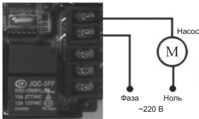
Рисунок 3-7. Подключение выхода сброса давления
