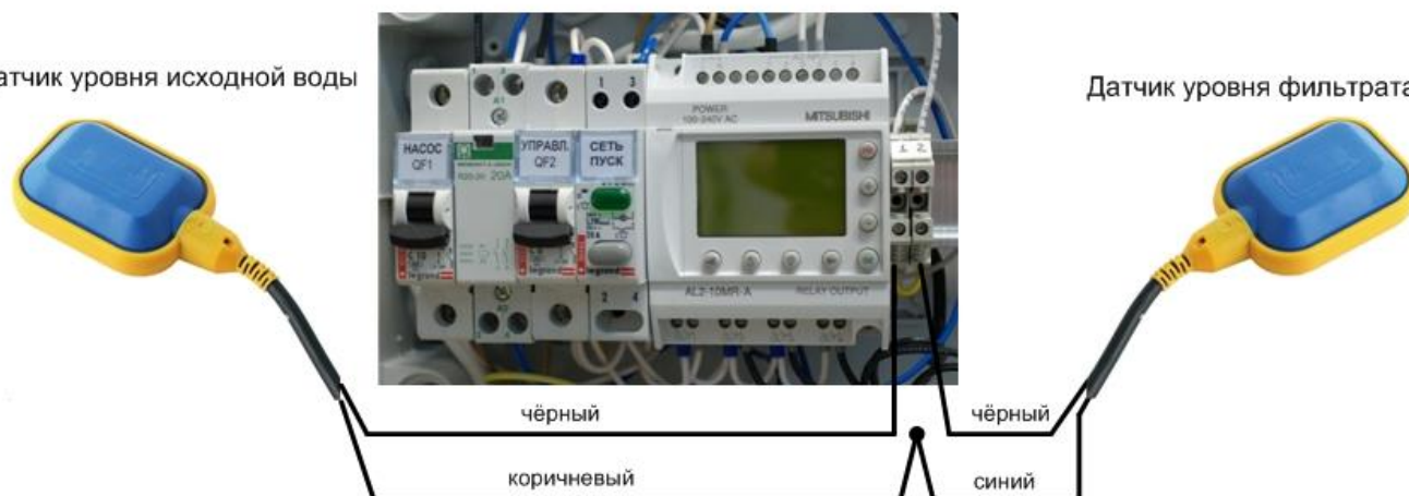
Блок управления RO-4040
