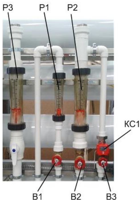
Рис.3 Ротаметры и вентили
