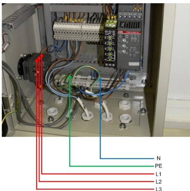
Рис.7 Подключение электропитания.
