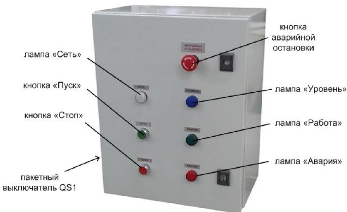
Рис.4 Блок управления.
