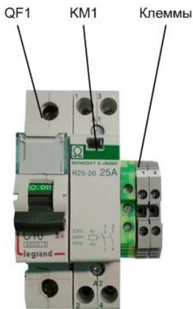
Рис.2 Элементы блока управления.
